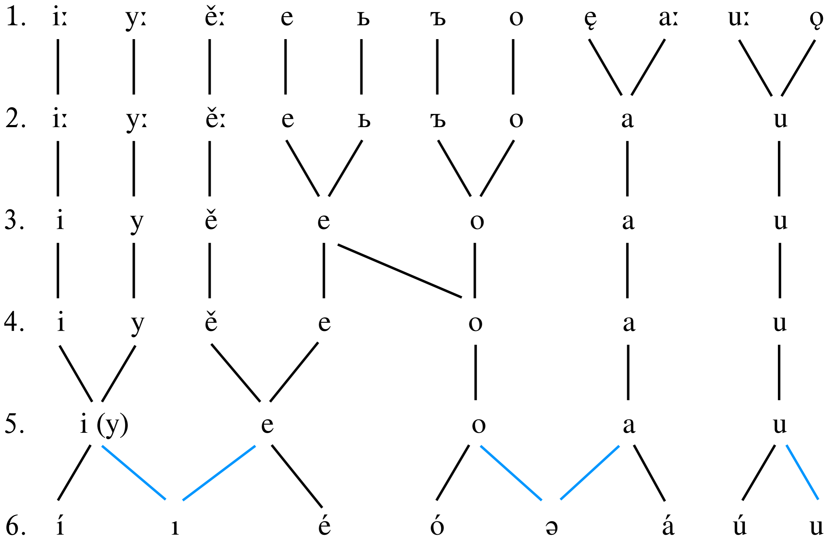
Reduktion + Akanje/Ikanje
